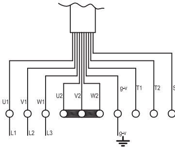
Électropompe avec câble à dix conducteurs: démarrage direct 400V Y
