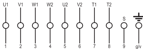
Câble à 10 conducteurs
