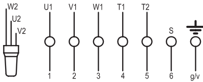
Câble à 7 conducteurs
