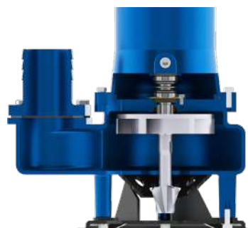
Vue en coupe d'une pompe GOVOX-S
