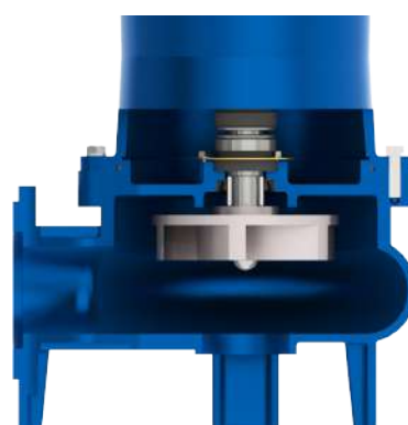
Vue en coupe d'une pompe GOVOX
