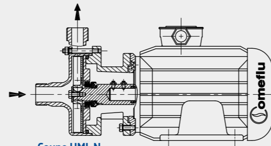
Coupe HMI-N avec garniture mécanique
