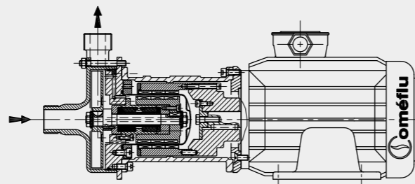
Coupe IMA avec entraînement magnétique
